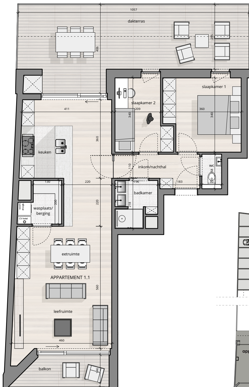
appartement verdieping 1 1.1
