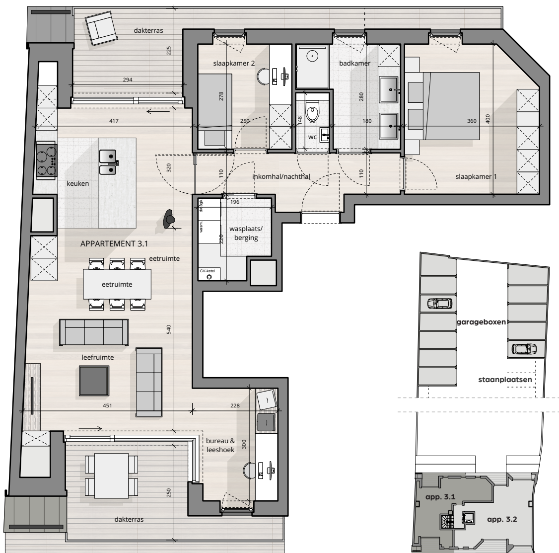
appartement verdieping 3 3.1
