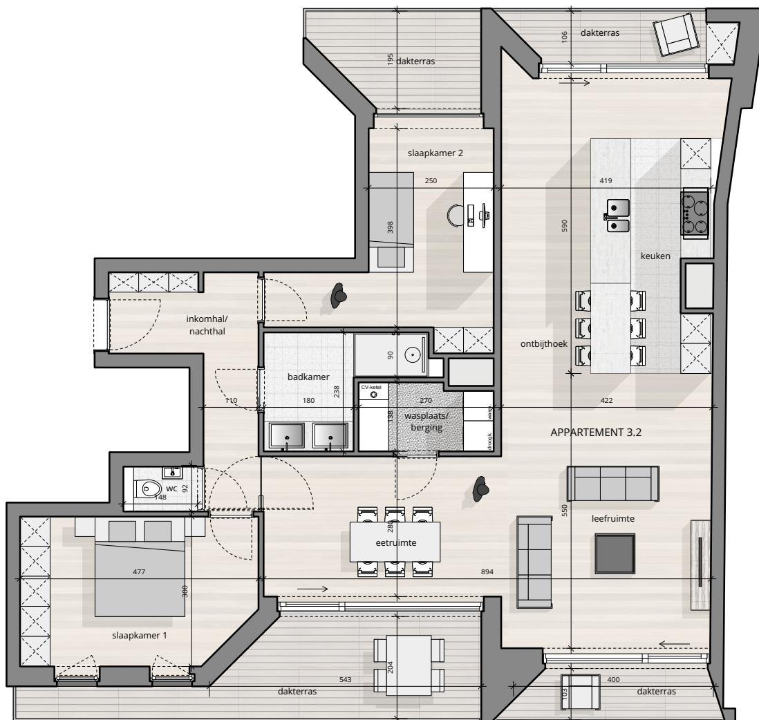
appartement verdieping 3 3.2
