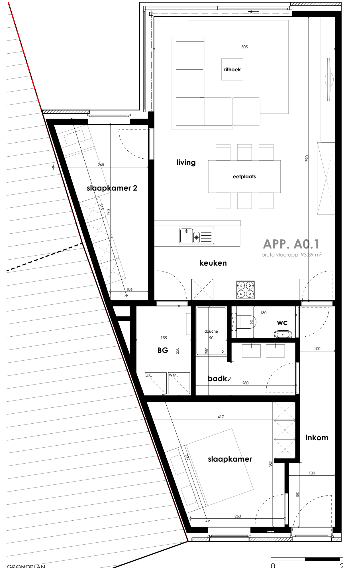
GRONDPLAN
