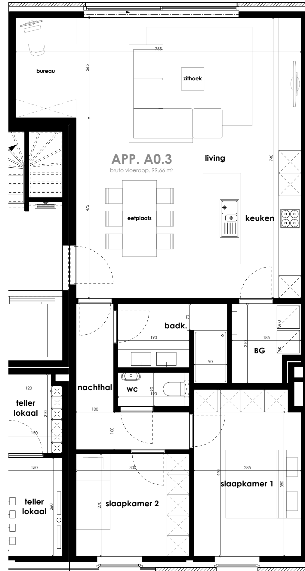
GRONDPLAN
