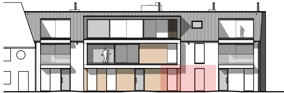
VOORGEVEL
