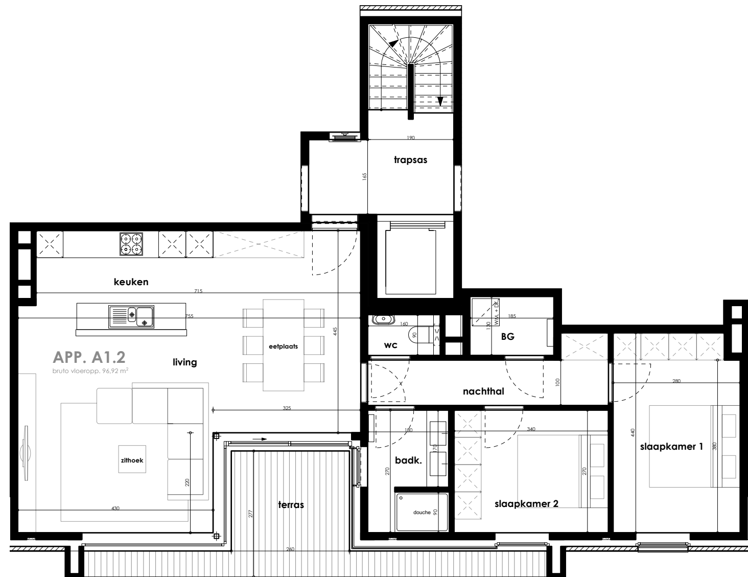
GRONDPLAN
