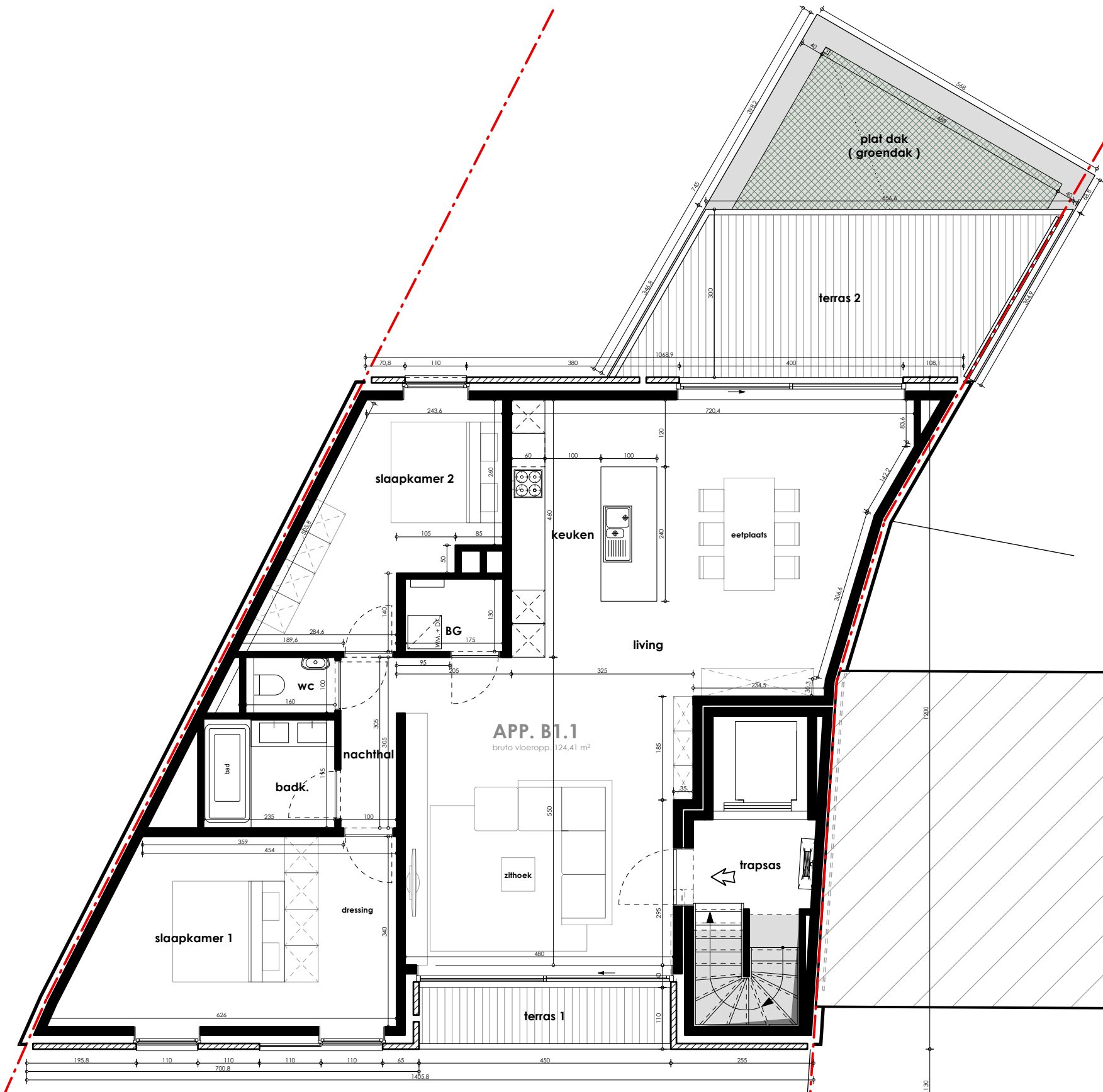
GRONDPLAN
