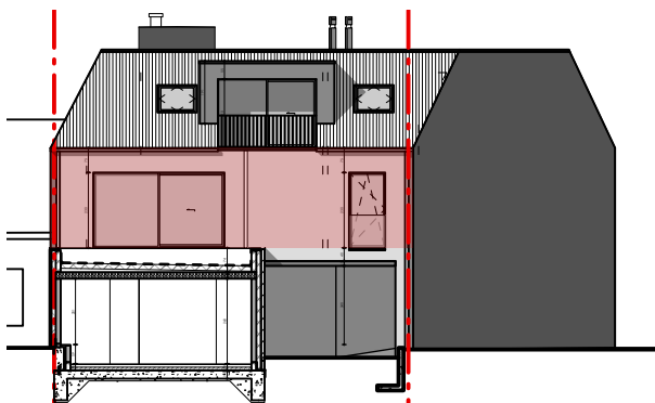
ACHTERGEVEL
